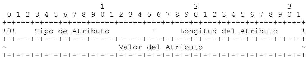
Figura 4a: Formato de los Atributo de los Datos TLV
