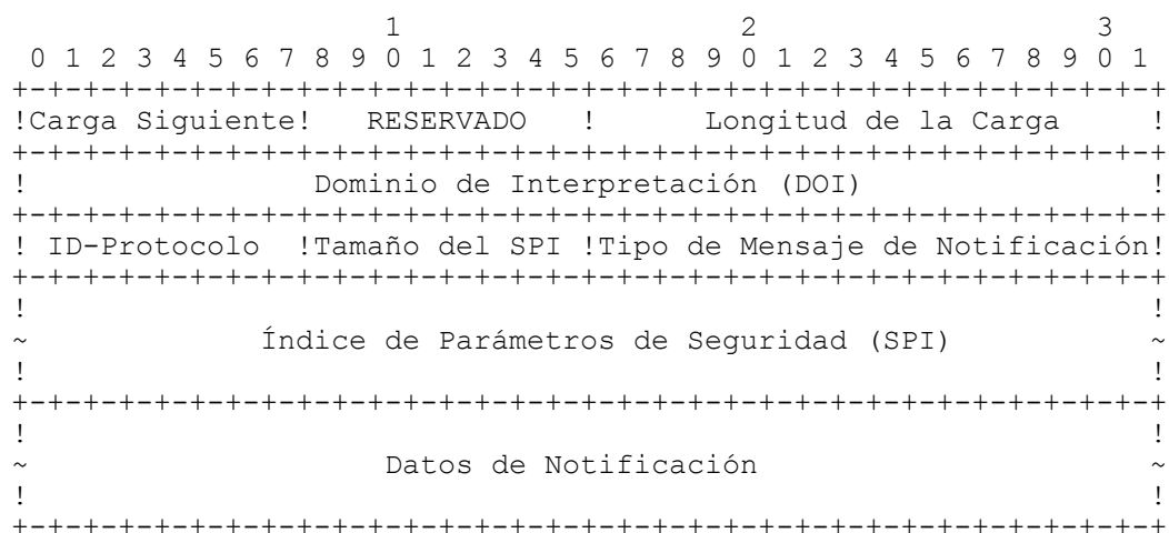
Figura 15: Formato de la Carga de Notificación
