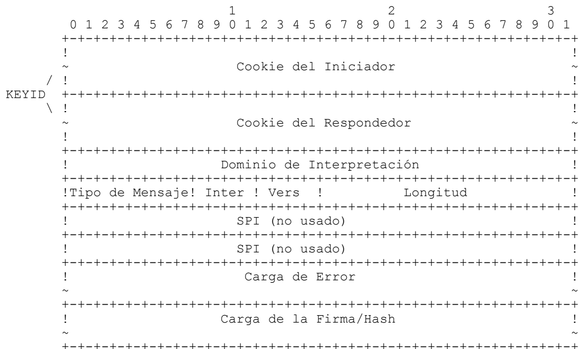
Figura 1: Mensaje de error de Oakley
