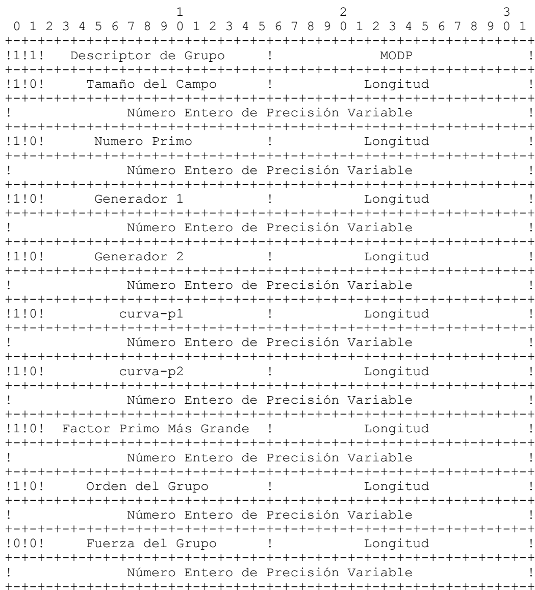
Figura 3: Ejemplo del formato un descriptor de grupo tipo MOD
