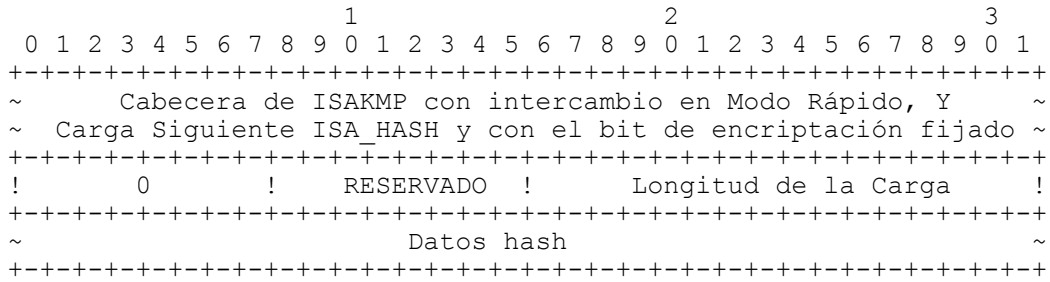
Figura 5: Cargas intercambiadas durante el Segundo intercambio de la Fase 2.
