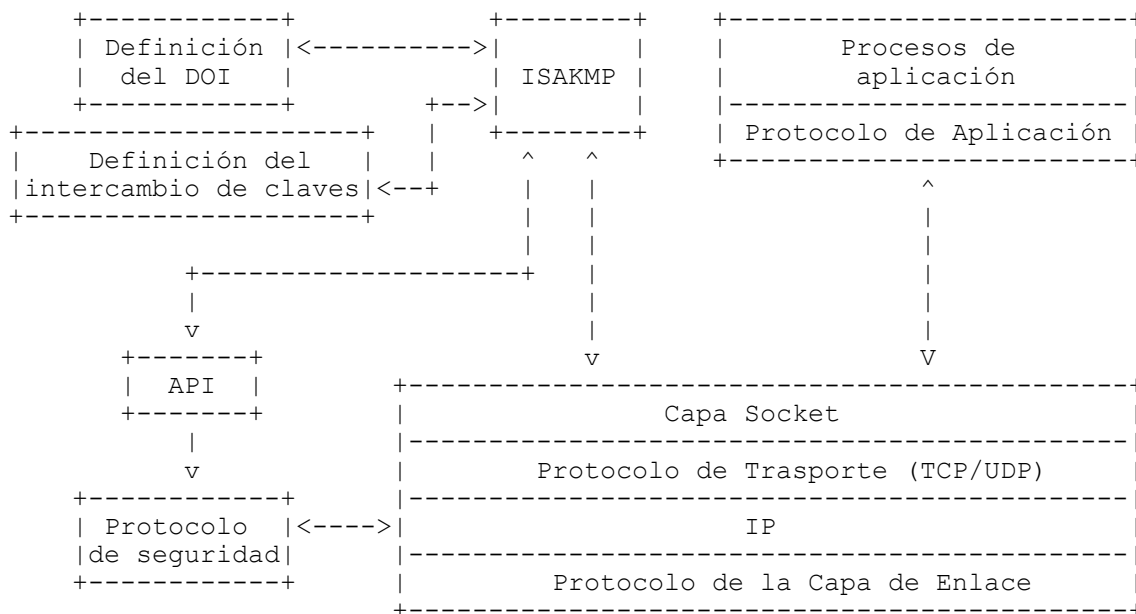
Figura 1: Ubicación de ISAKMP
