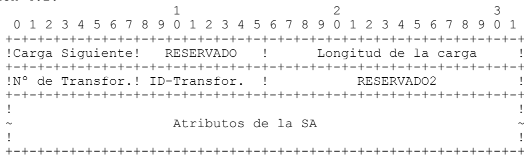
Figura 7: Formato de la Carga de Transformación
