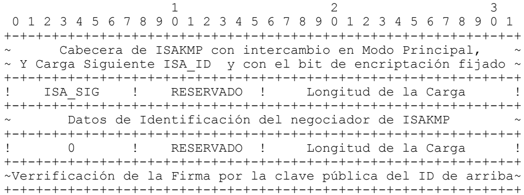
Figura 3: Cargas intercambiadas durante el tercer intercambio de la Fase 1 utilizando el Modo Principal.
