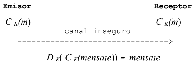
Figura 1: Sistemas de clave privada o simétricos
