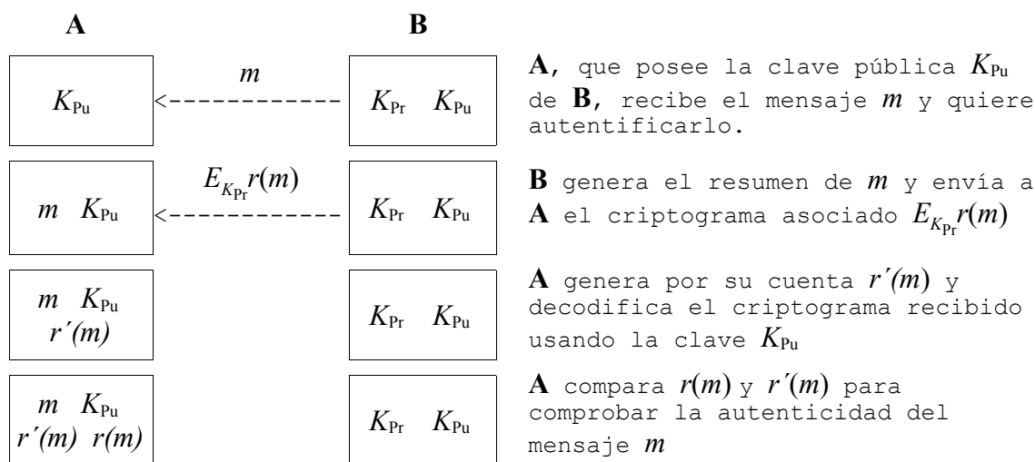
Figura 5: Autenticación de la información empleando algoritmos asimétricos.
