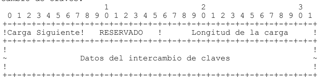
Figura 8: Formato de la Carga de Intercambio de Claves
