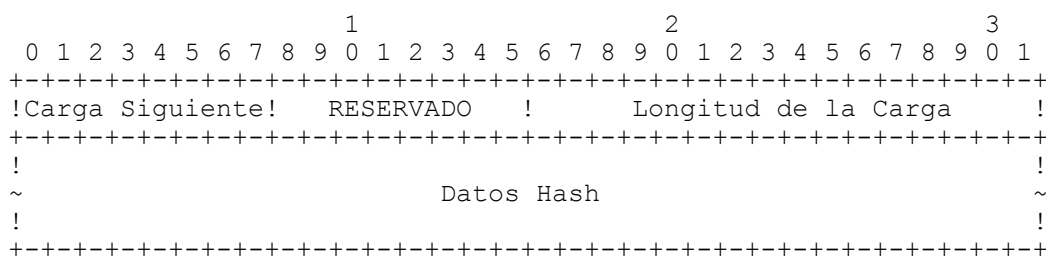
Figura 12: Formato de la carga Hash.
